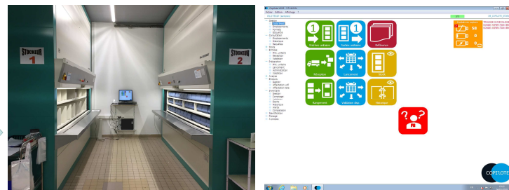
Installation 2 Stockeurs Rotatifs et du logiciel de gestion de stock Copilote
